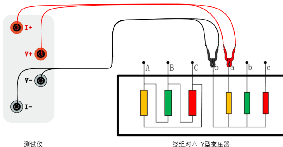
图 2 常规 Y 型单相测量法接线图
