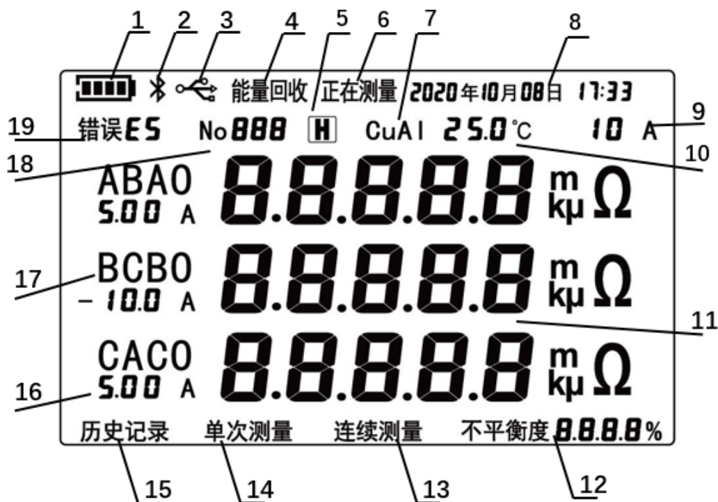
图 1 OLED 液晶屏幕布局
