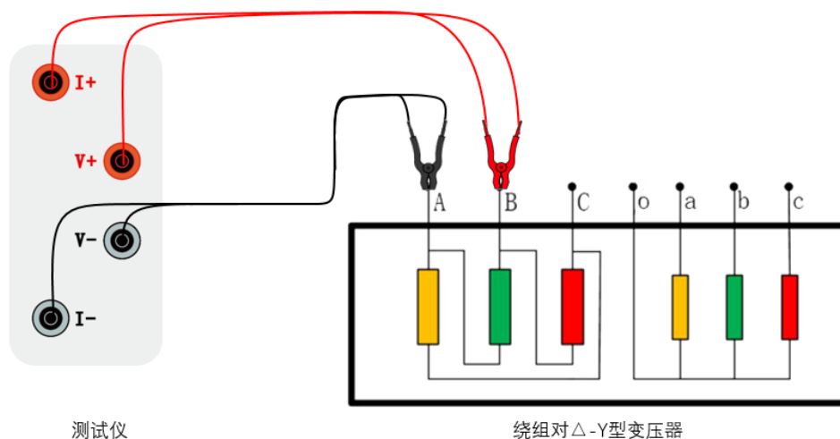
图 3 常规 \Delta 型单相测量法接线图
